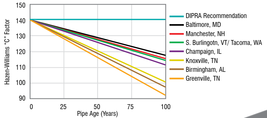
FIGURE 3: "C" VALUES FOR DI PIPE / DIPRA BROCHURE
